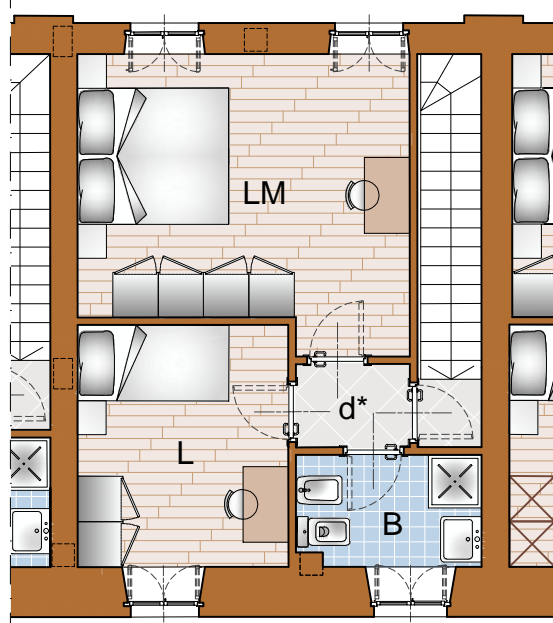
PIANO PRIMO
